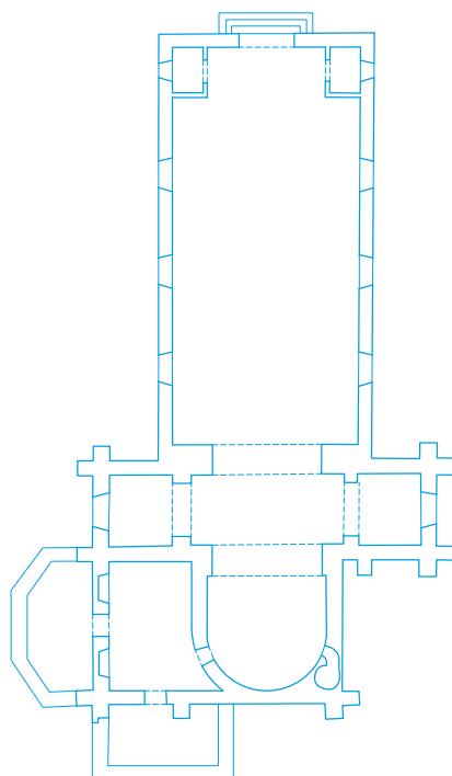
PLAN DE L'ÉGLISE RÉALISÉ EN 1817 PAR JACQUES MOLINOS
