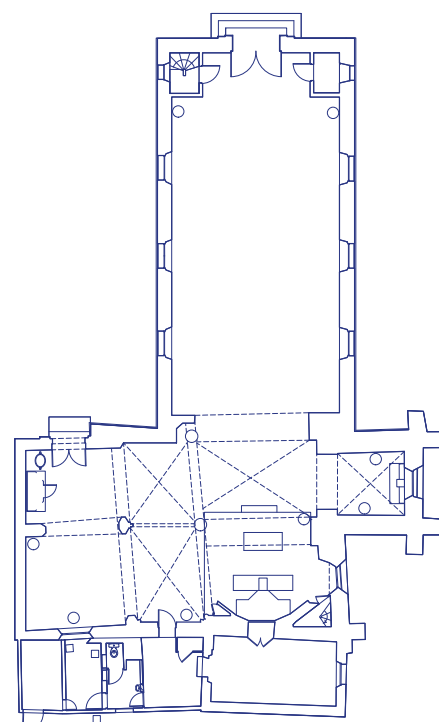
PLAN ACTUEL DE L'ÉGLISE
